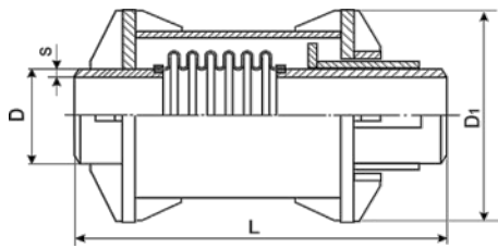
Основные параметры блочного компенсатора односильфонного / двухсильфонного осевого типа КСО
