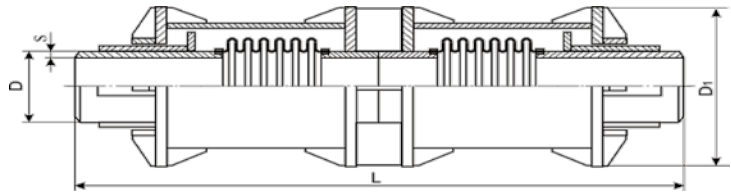
Основные параметры блочного компенсатора односильфонного / двухсильфонного осевого типа КСО
