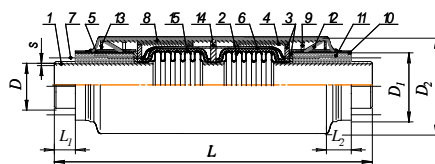
Основные параметры устройства односильфонного и двухсильфонного компенсационного типа SKU.PPU/PU.II XXX* - материал патрубка компенсатора
