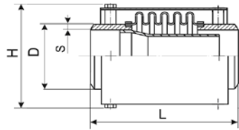
Общий вид компенсатора односильфонного осевого с патрубками под приварку с наружным кожухом и направляющим экраном типа ОПМ
