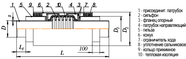
Основные параметры устройства односильфонного и двухсильфонного компенсационного типа SKU.PPM XXX* - материал патрубка компенсатора
