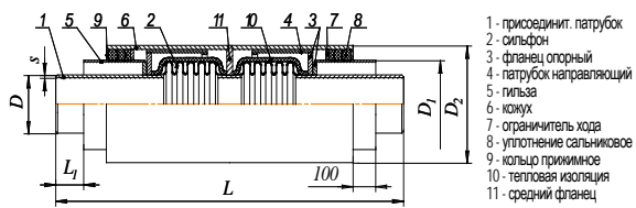
Основные параметры устройства односильфонного и двухсильфонного компенсационного типа SKU.PPM XXX* - материал патрубка компенсатора
