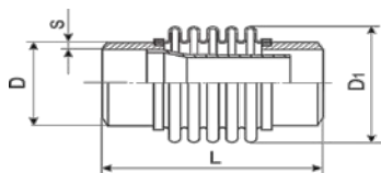
Общий вид компенсатора односильфонного осевого с патрубками под приварку с внутренним направляющим экраном типа ОПГ
