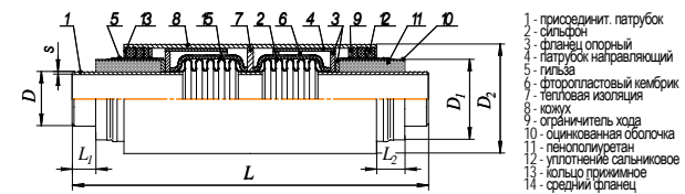
Основные параметры устройства односильфонного и двухсильфонного компенсационного типа SKU. ППУ. ОЦ XXX* - материал патрубка компенсатора
