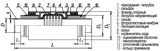
Основные параметры устройства односильфонного и двухсильфонного компенсационного типа SKU. ППУ. ОЦ XXX* - материал патрубка компенсатора
