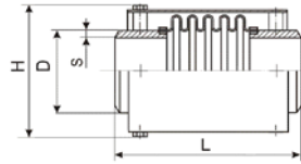
Общий вид компенсатора односильфонного осевого с патрубками под приварку с наружным кожухом типа ОПК
