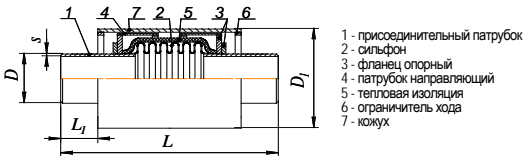
Основные параметры устройства односифонного и двухсифонного компенсационного типа SKU.MП XXX* - материал патрубка компенсатора
