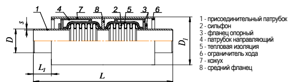
Основные параметры устройства односифонного и двухсифонного компенсационного типа SKU.MП XXX* - материал патрубка компенсатора
