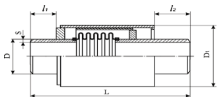
Общий вид компенсатора односифонного / двухсифонного осевого с патрубками под приварку с усиленным наружным кожухом типа ОПКР
