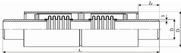
Общий вид компенсатора односифонного / двухсифонного осевого с патрубками под приварку с усиленным наружным кожухом типа ОПКР
